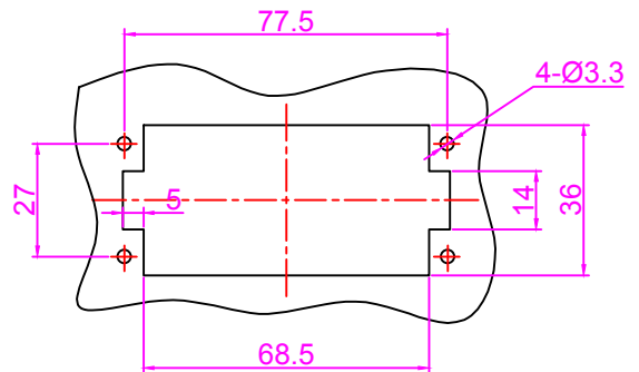
面板开孔图 Panel cut
