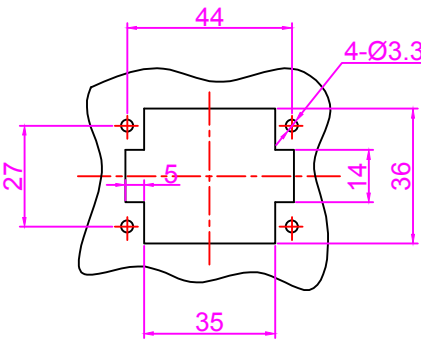
面板开孔图 Panel cut
